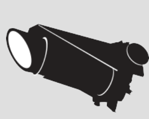
K2
