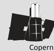
Copernicus
