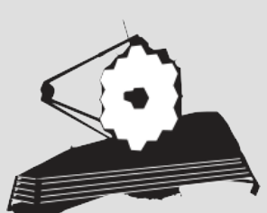
JWST
